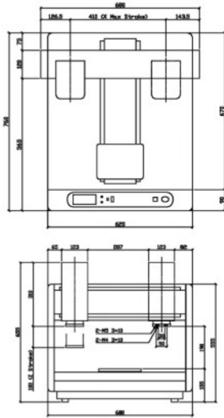
I&J7400 dimensions
